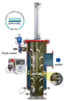
FTAF Bernoulli
